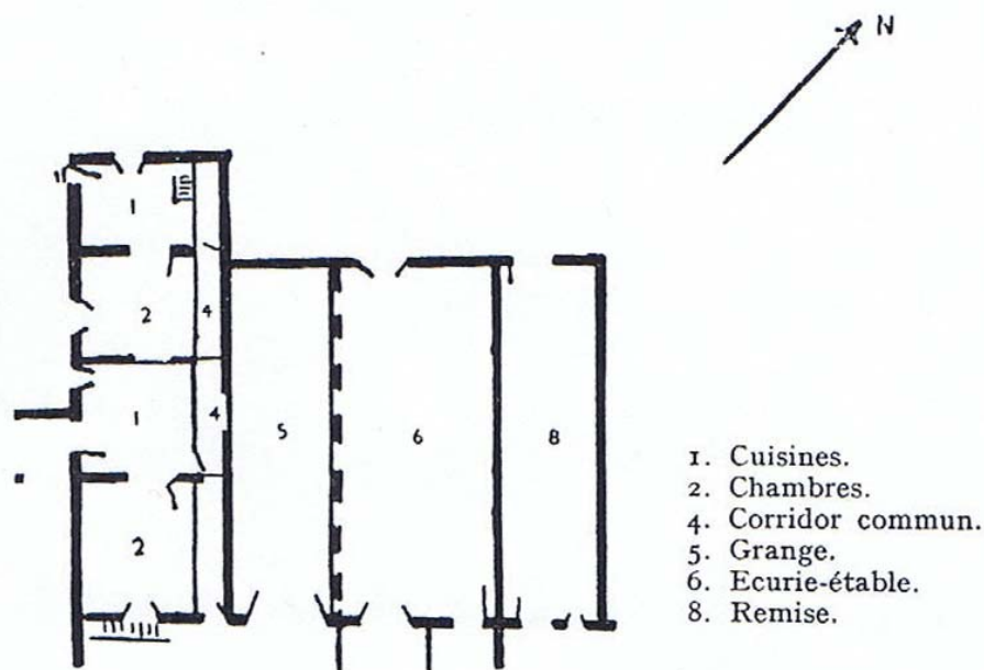
MAISON A LA RUSSILLE (LES CLÉES) Division longitudinale.
