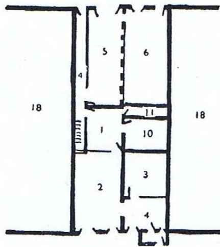
MAISON DU VILLAGE DU LIEU bâtie en contiguïté, division longitudinale.
